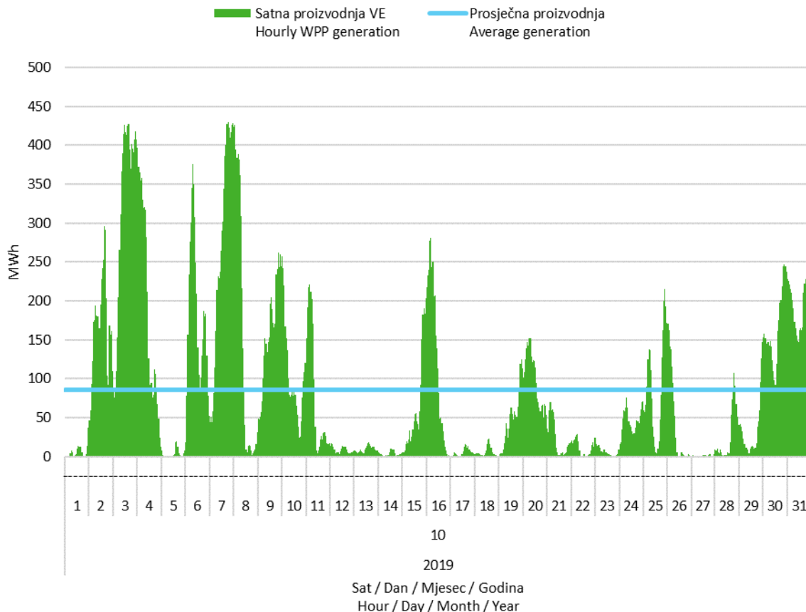
Slika 2 Satna proizvodnja svih vjetroelektrana u listopadu 2019. godine
