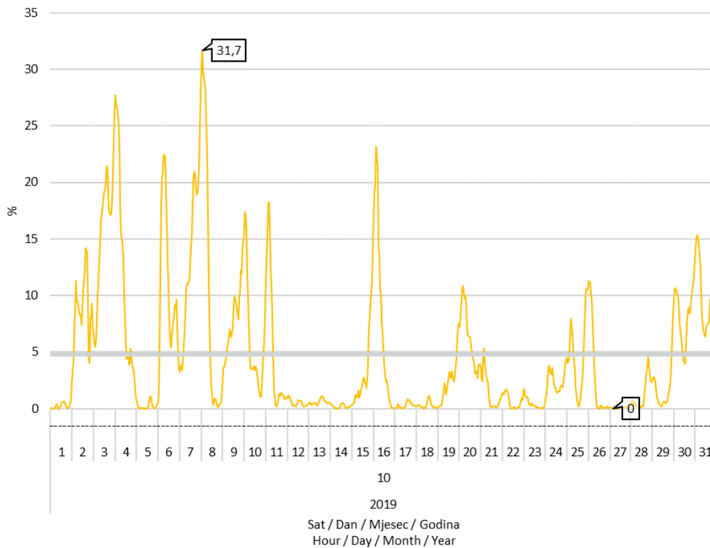
Slika 8 Udio proizvodnje vjetroelektrana u pokrivanju satnog opterećenja elektroenergetskog sustava u listopadu 2019. godine
