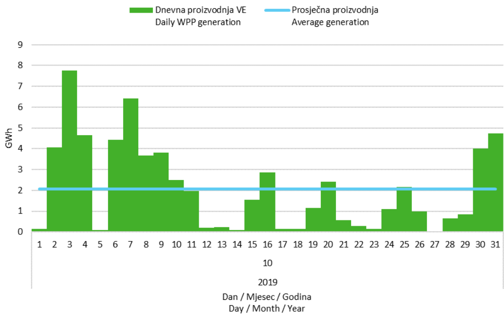
Slika 5 Dnevna proizvodnja svih vjetroelektrana u listopadu 2019. godine Figure 5 Daily generation of all wind power plants in October 2019
