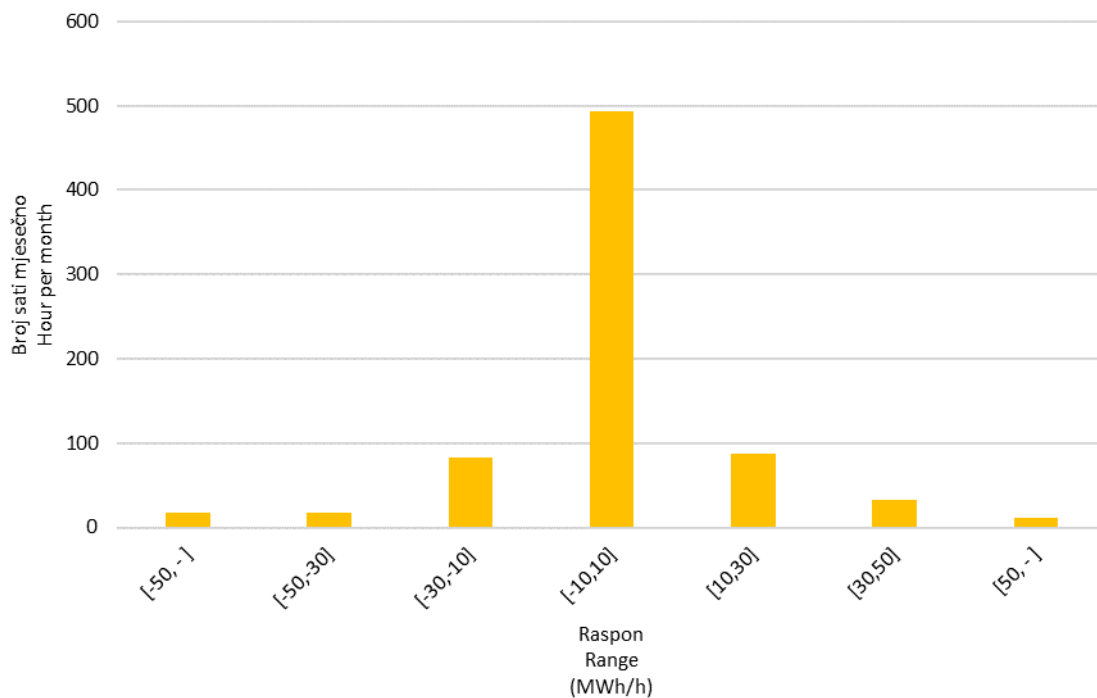
Slika 10 Statistička raspodjela satnih promjena proizvodnje VE u listopadu 2019. godine
