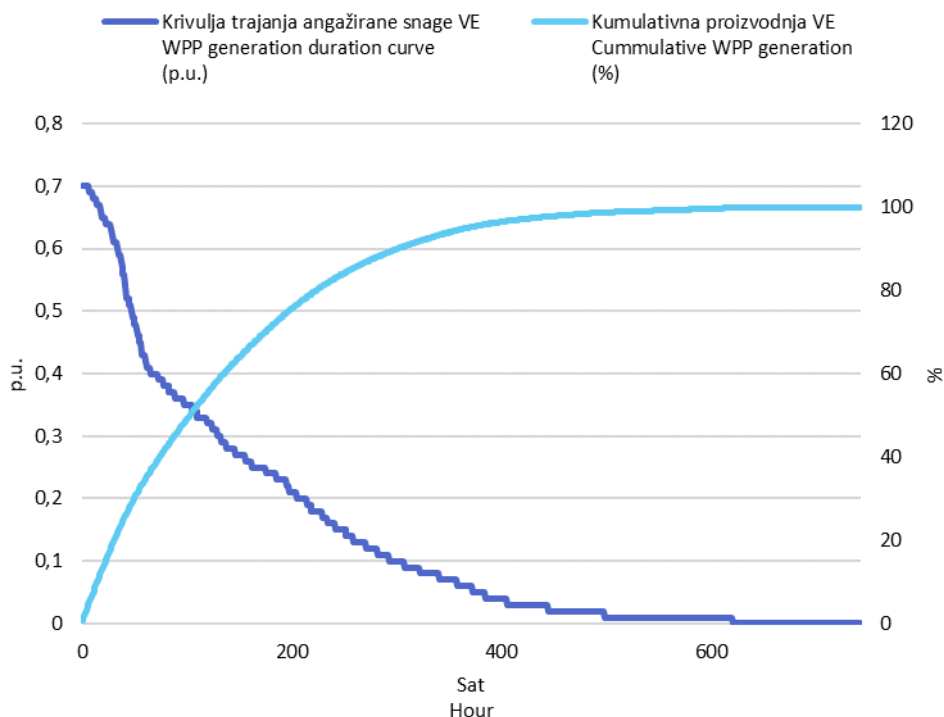
Slika 3 Krivulja trajanja angažirane snage svih VE i kumulativna proizvodnja VE u listopadu 2019. godine u jediničnim vrijednostima
