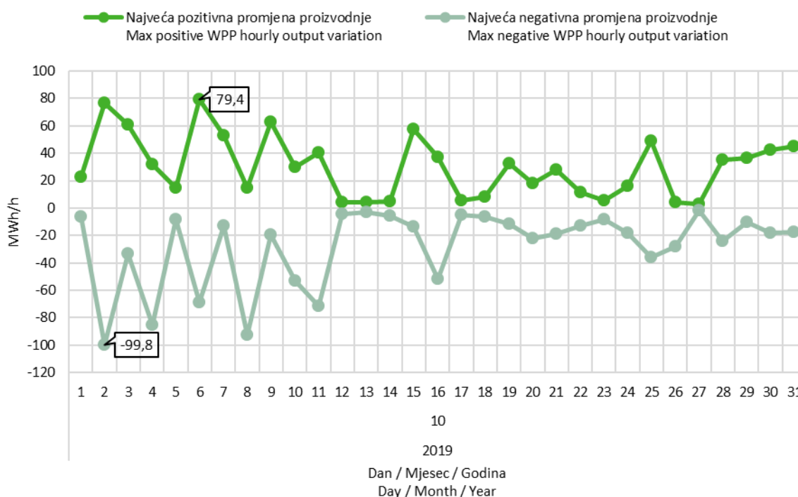
Slika 9 Maksimalna pozitivna i maksimalna negativna promjena satne proizvodnje VE u listopadu 2019. godine
