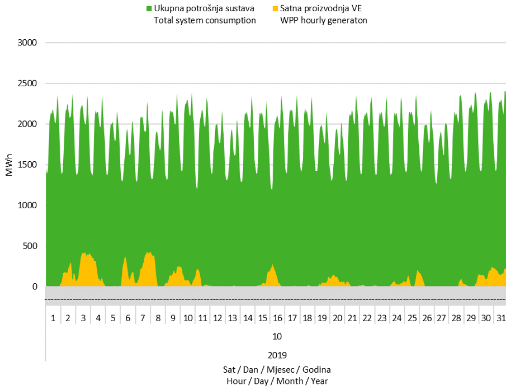
Slika 7 Usporedba satnog dijagrama opterećenja sustava i proizvodnje vjetroelektrana u listopadu 2019. godine
