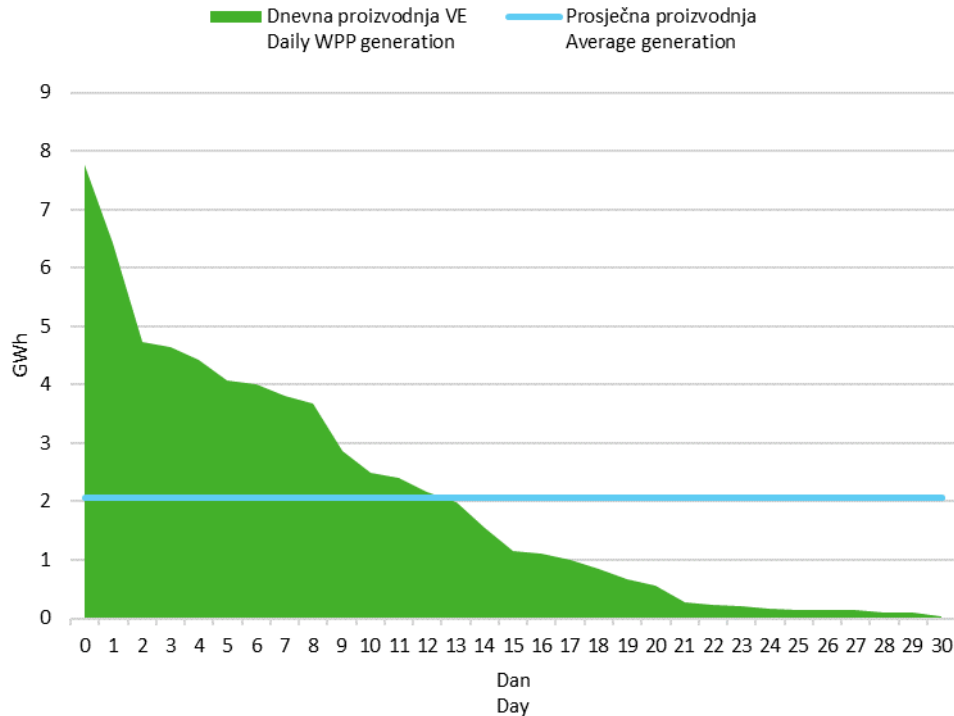
Slika 6 Krivulja trajanja dnevne proizvodnje vjetroelektrana u listopadu 2019. godine
